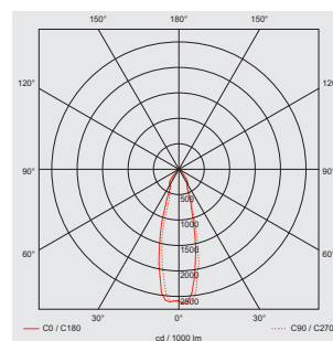
Angle de rayonnement 24°
